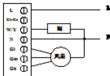
VC4043 阀接线图
