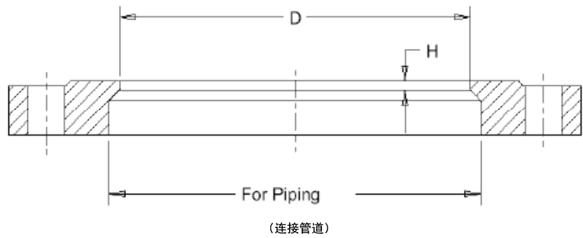
法兰规格（中线蝶阀法兰）
