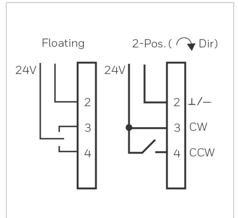
开关型: MVN6105../MVN6110..
